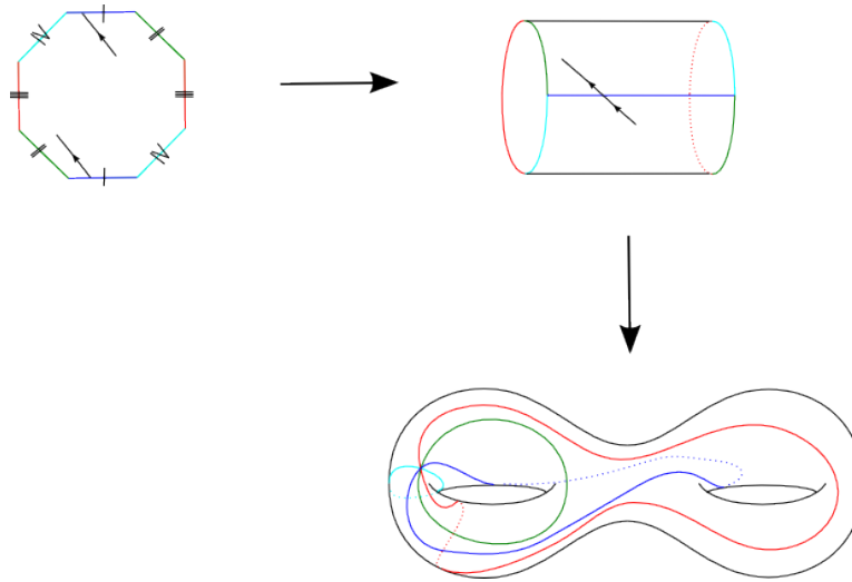
ABBILDUNG 2. Kegelwinkel 4\pi
