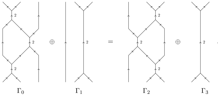
Figure 4: Eine MOY-Relation
