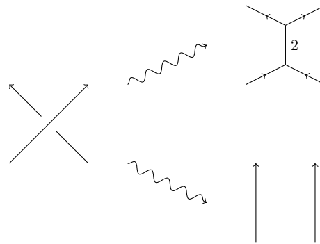
Figure 1: Auflösen einer Überkreuzung
