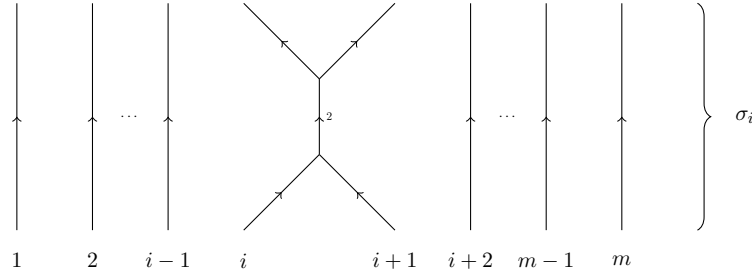
Figure 3: Baustein \sigma_i eines MOY-Zopfes
