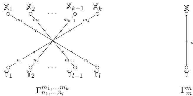
Figure 2: Einfache MOY-Graphen
