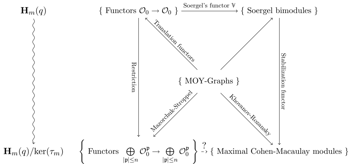
Figure 5: Überblick über die Ergebnisse dieser Arbeit
