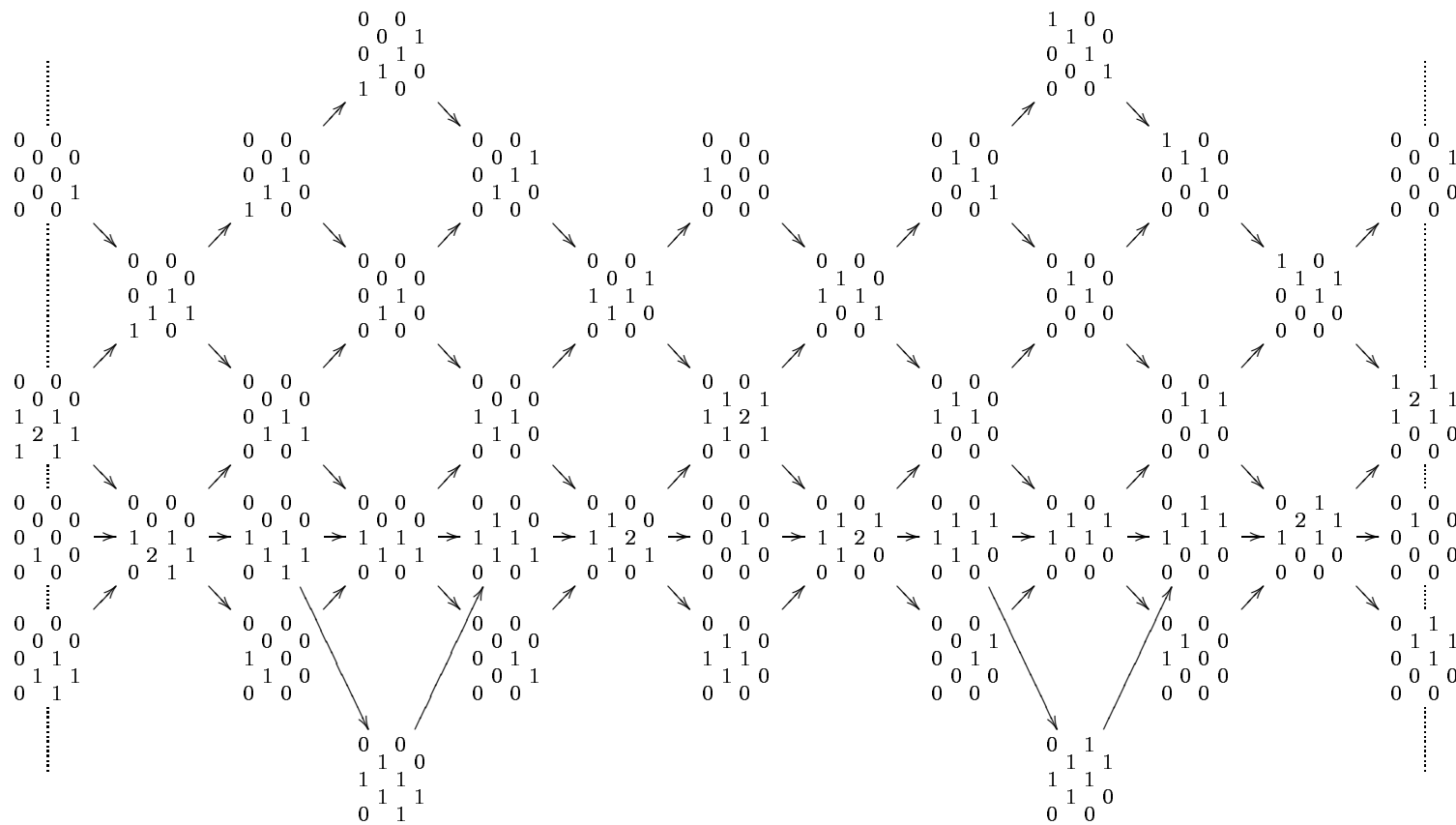
The Auslander-Reiten quiver of \Lambda_4
